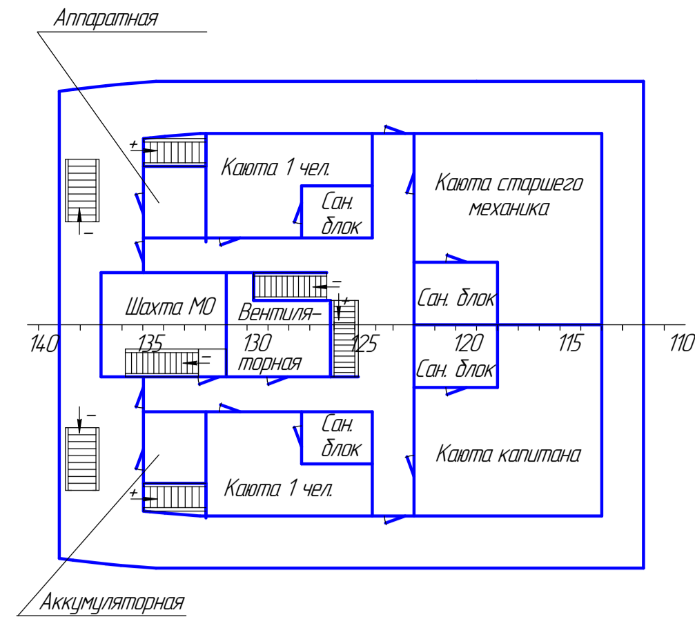
Палуба рубки 1 яруса
