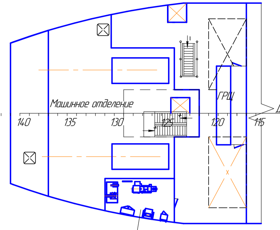
Платформа в МО
