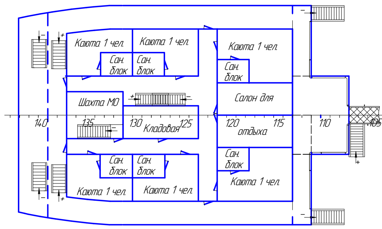
Палуба надстройки
