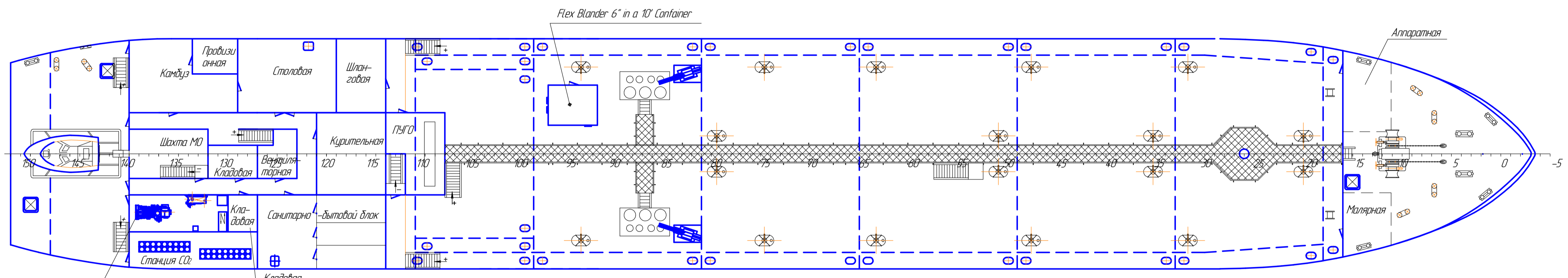
Верхняя палуба
