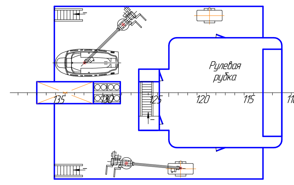
Палуба рубки 2 яруса
