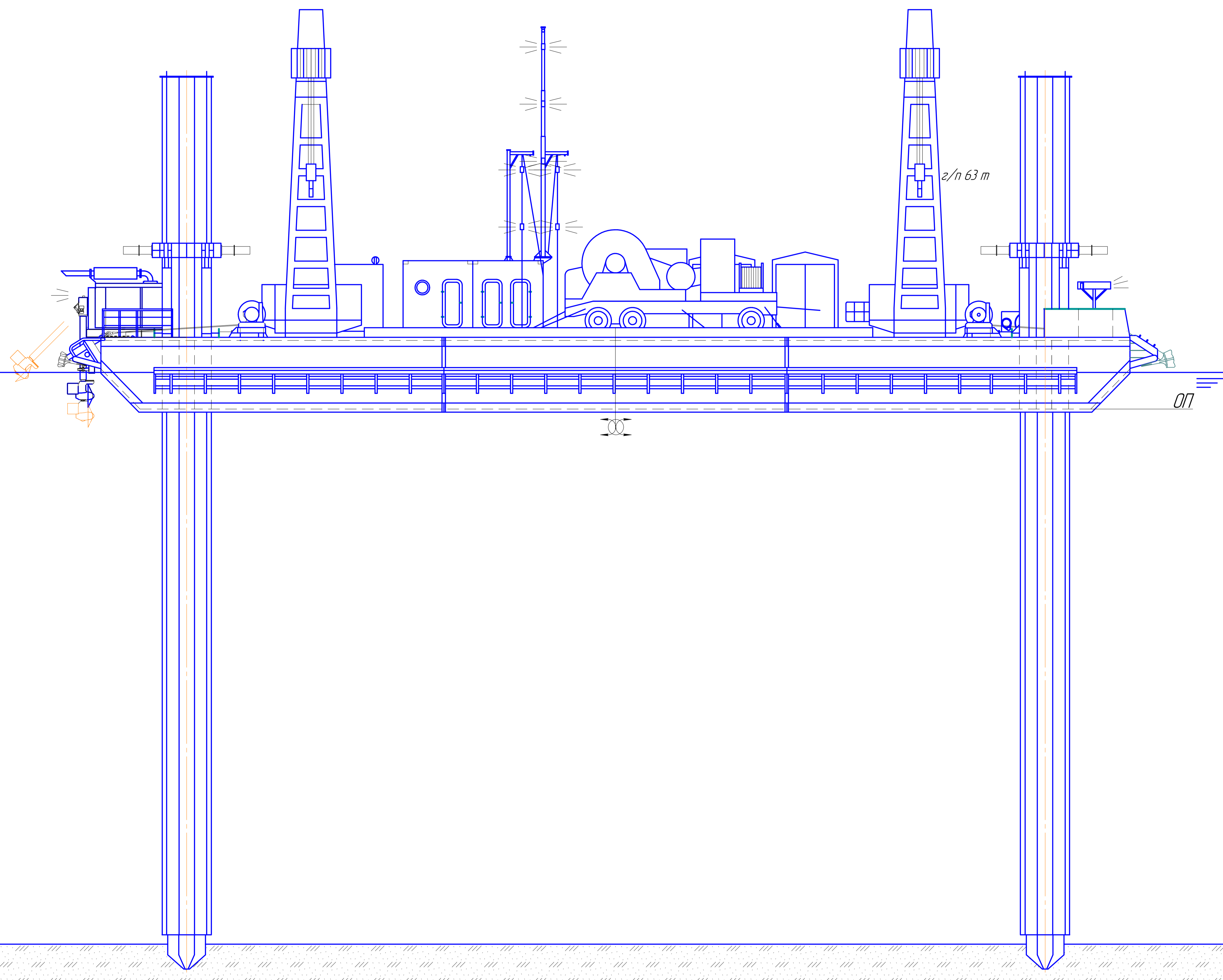
Боковой вид
