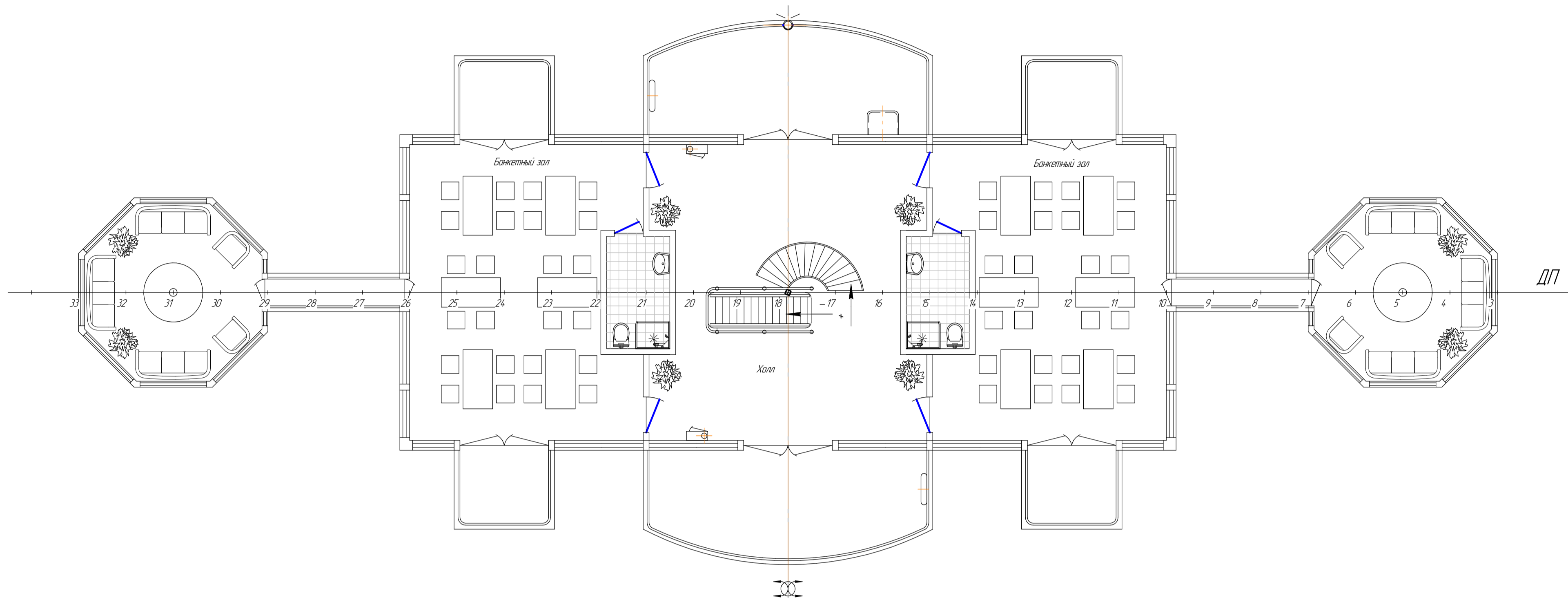
Палуба надстройки первого яруса
