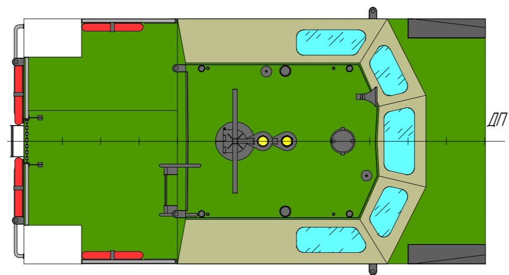
Крыша пассажирской рубки
