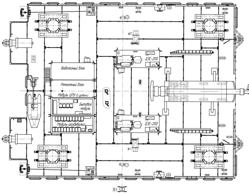
Вид сверху
