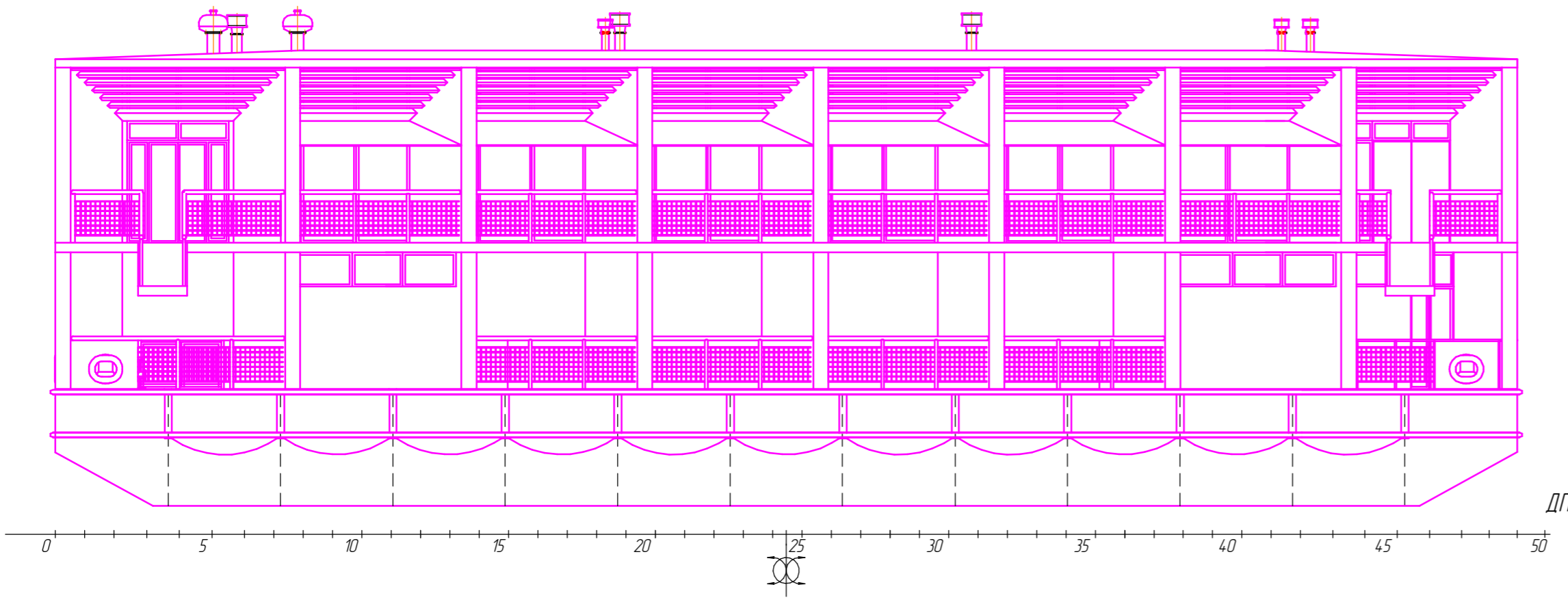
Левый борт
