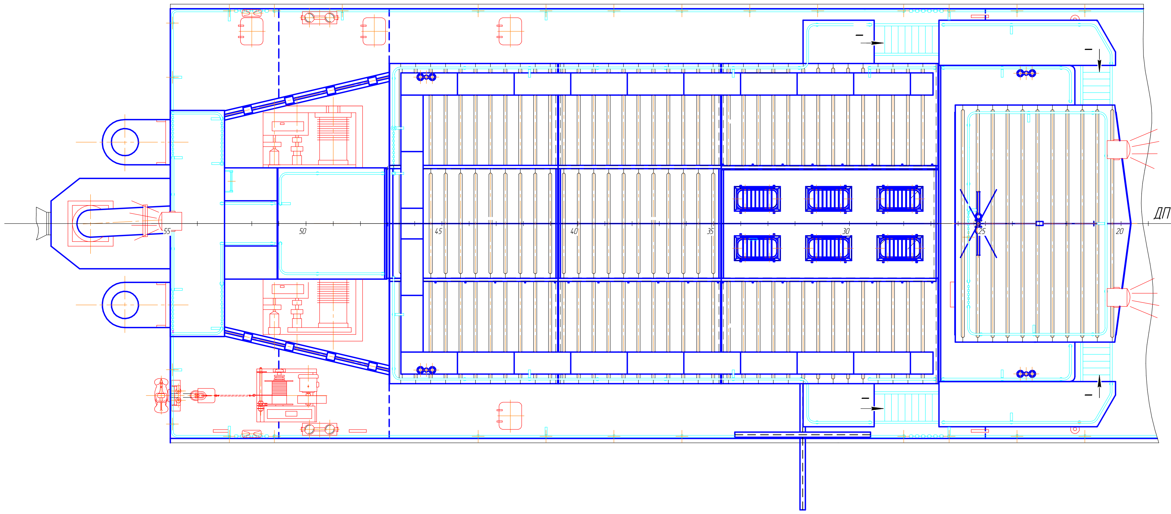
План расположения оборудования в машинном зале и в трюмах
