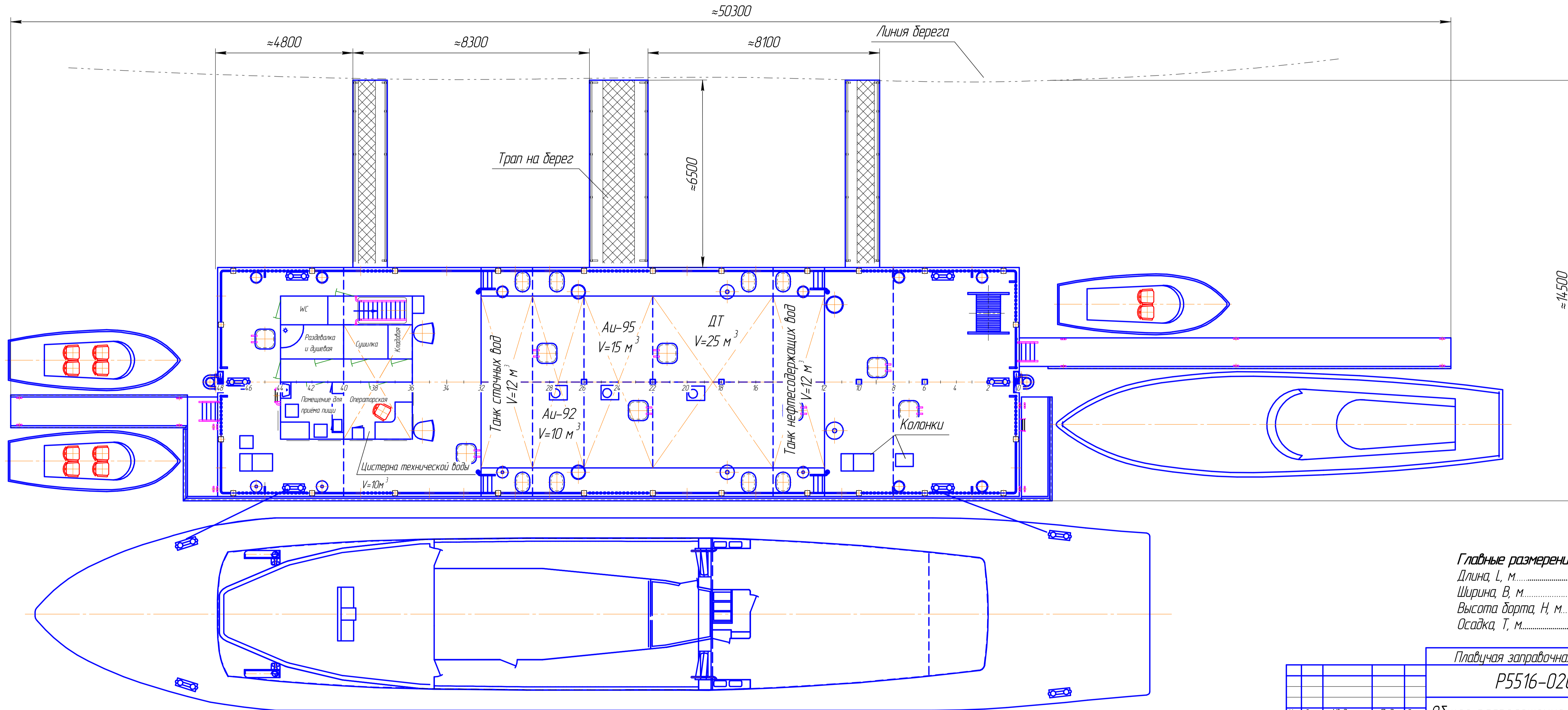
Вид сверху (при снятой тентовой палубе)
