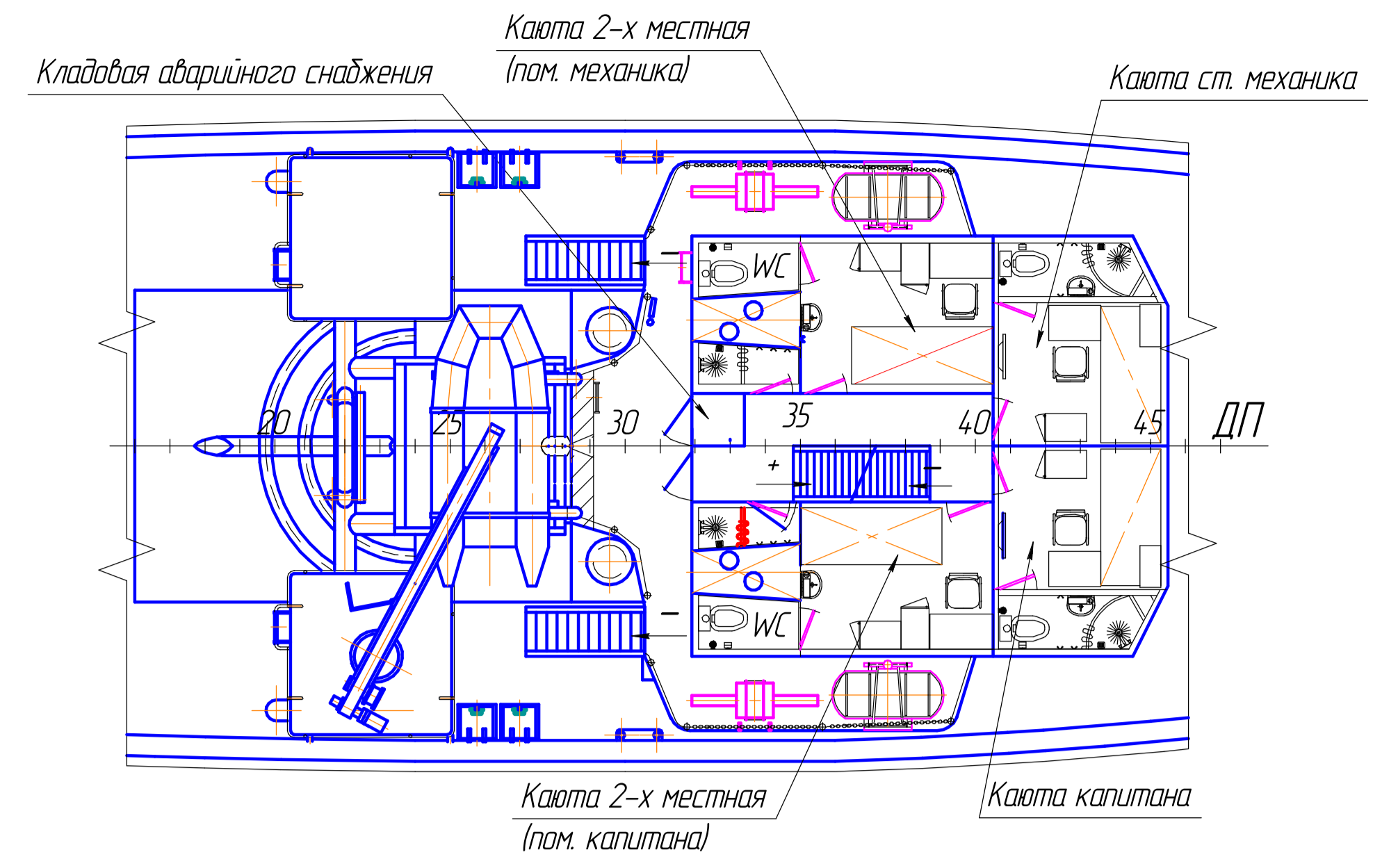
Палуба рубки 1-ого яруса
