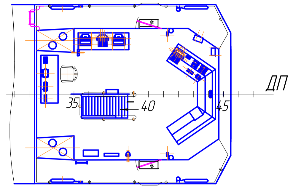
Палуба рубки управления
