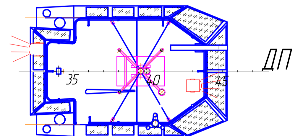
Палуба рубки управления
