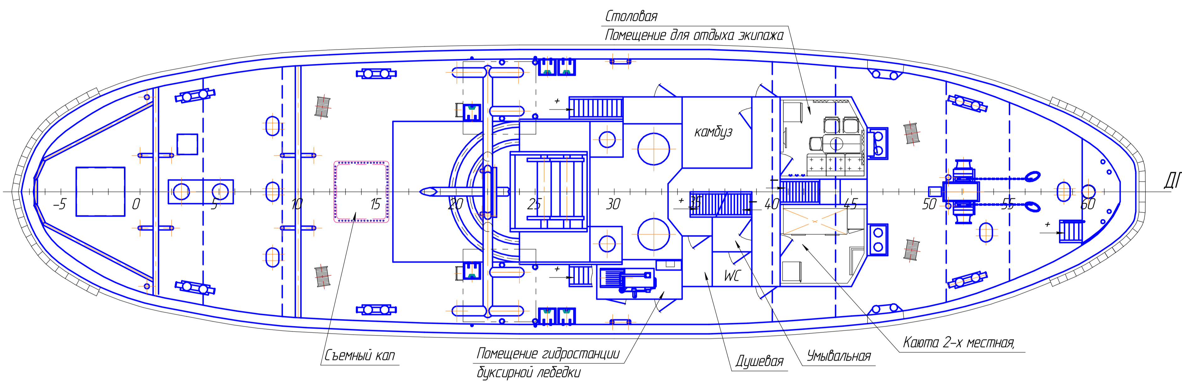
Главная палуба
