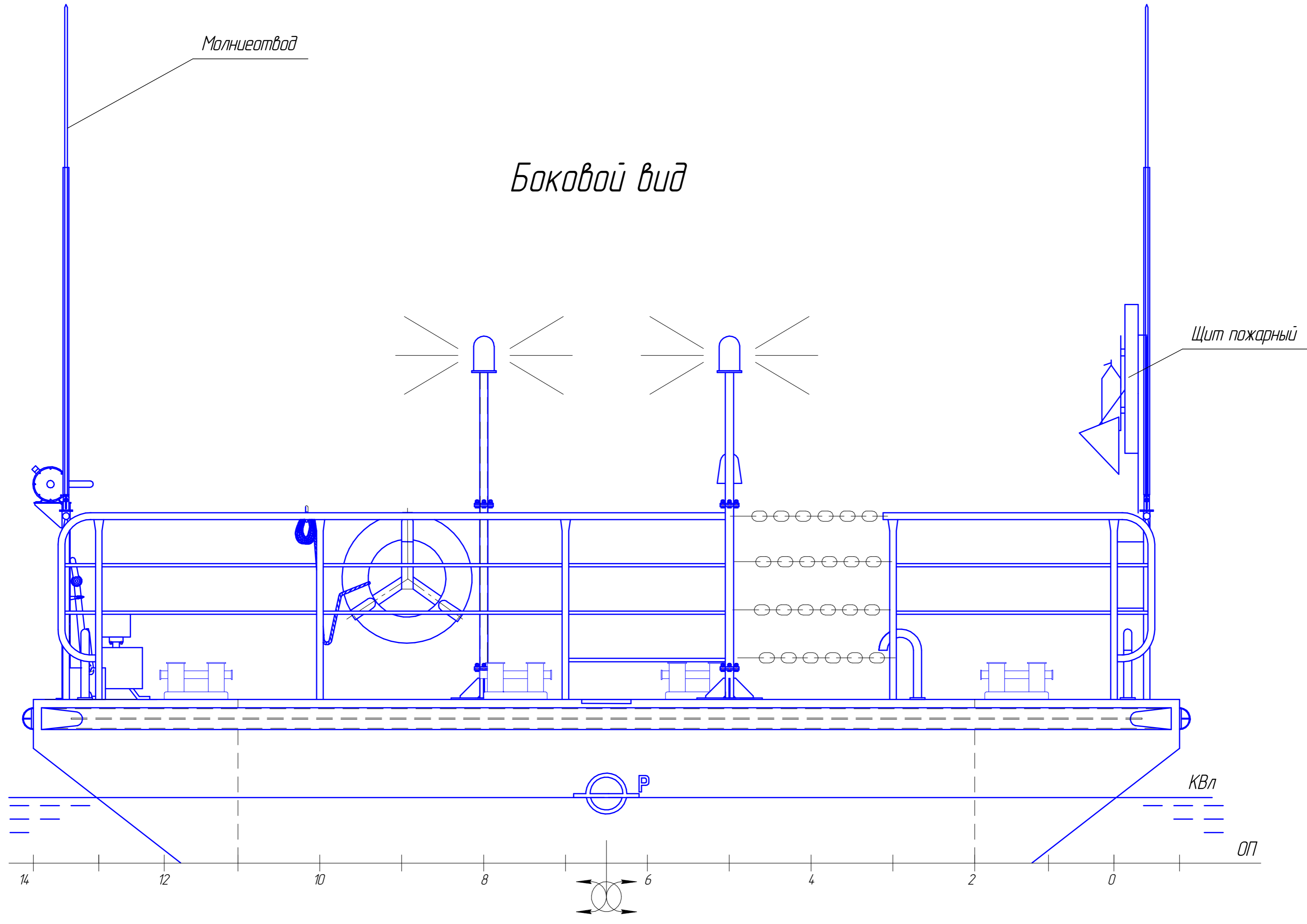
Боковой вид
