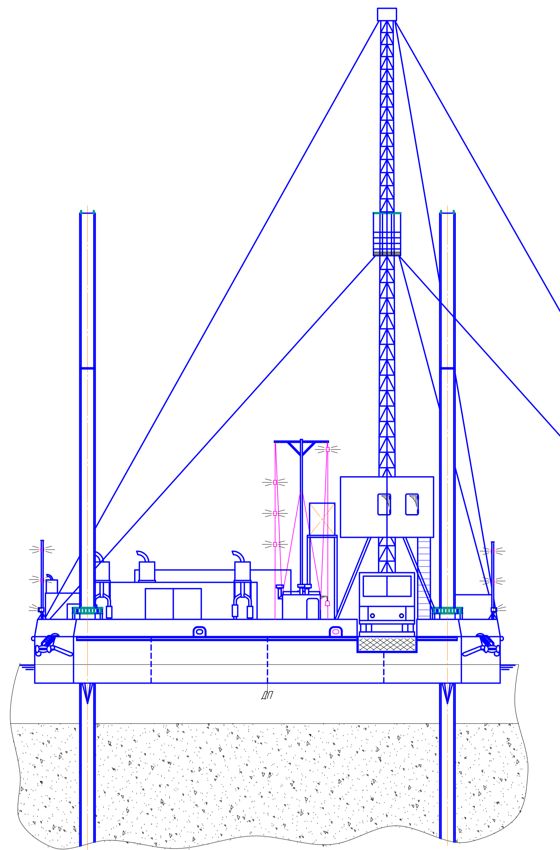
Вид в нос
