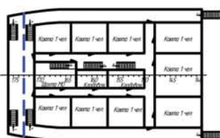
Палуба надстройки
