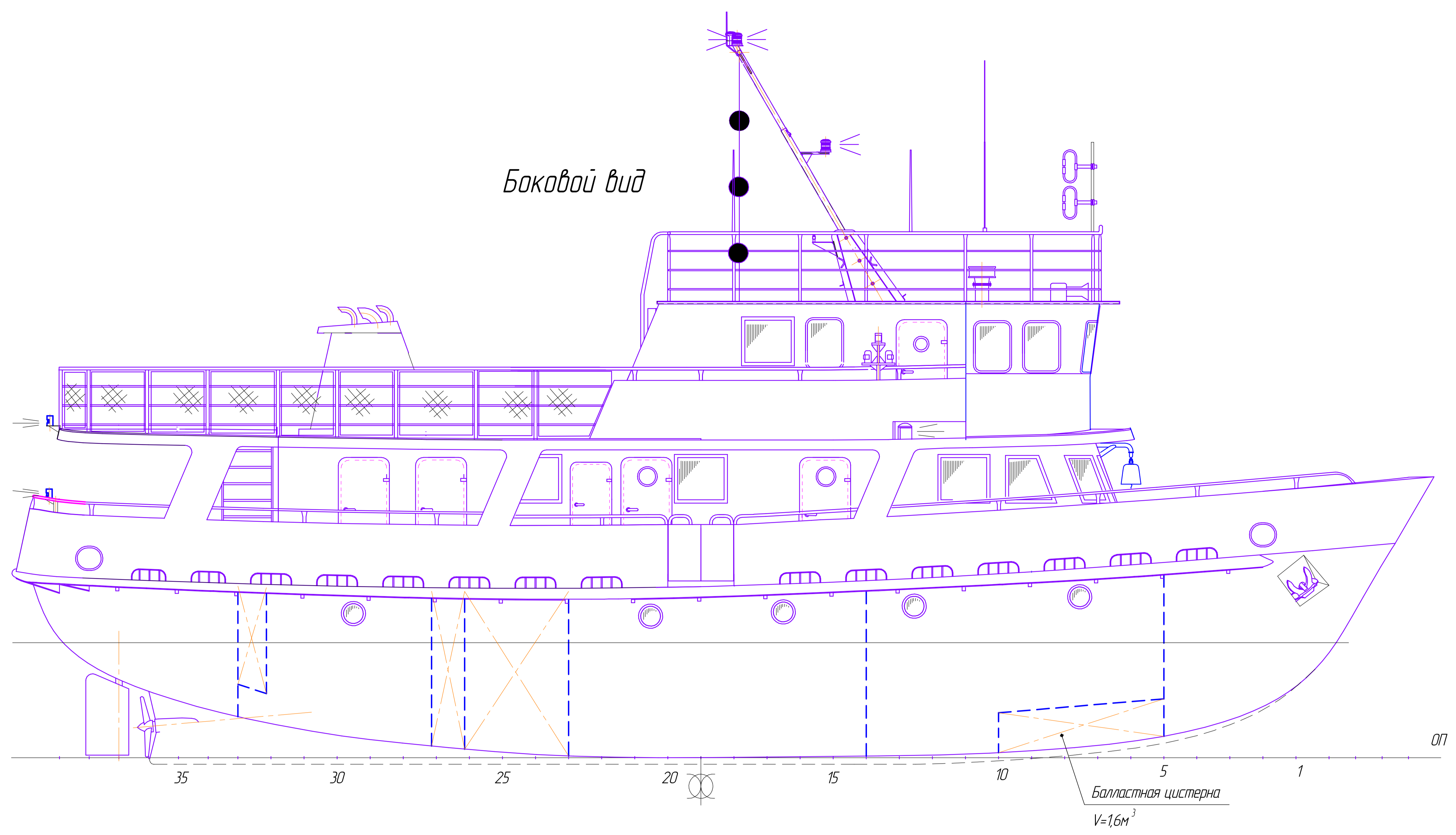
Боковой вид
