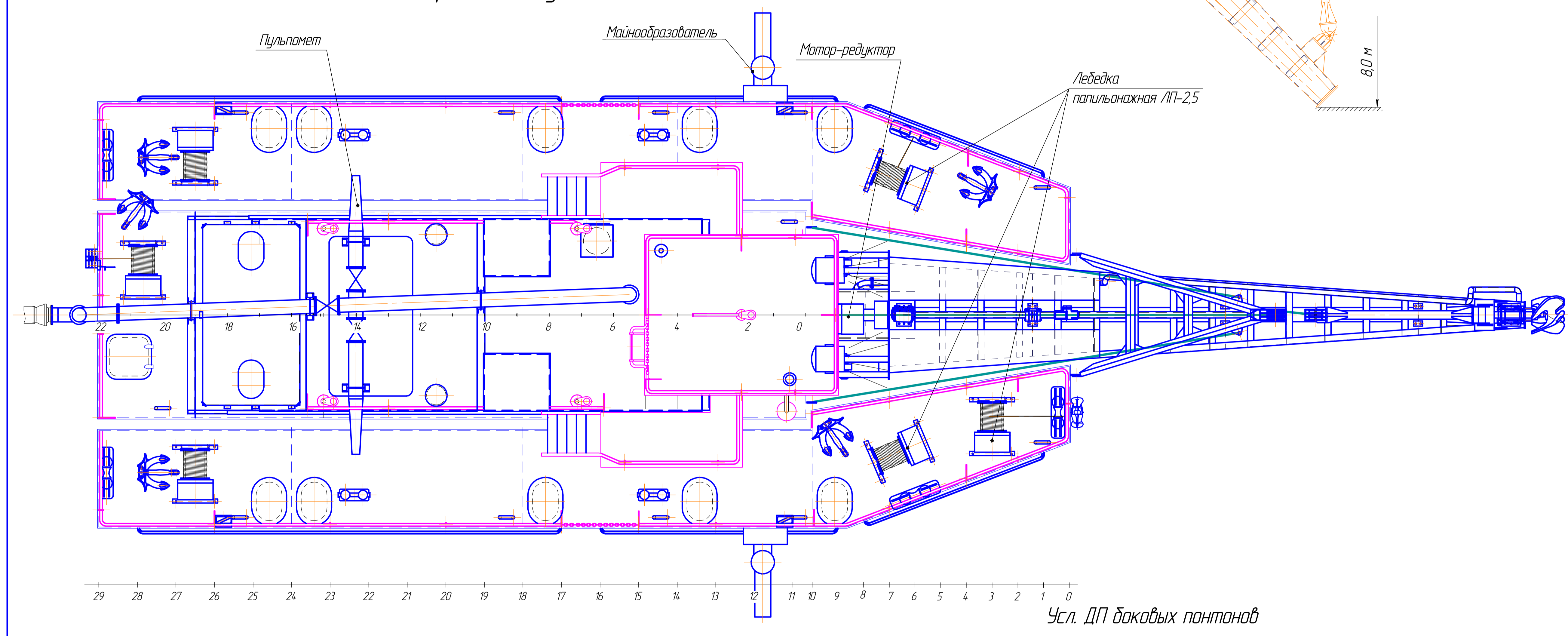
Вид сверху (со снятой рубкой)
